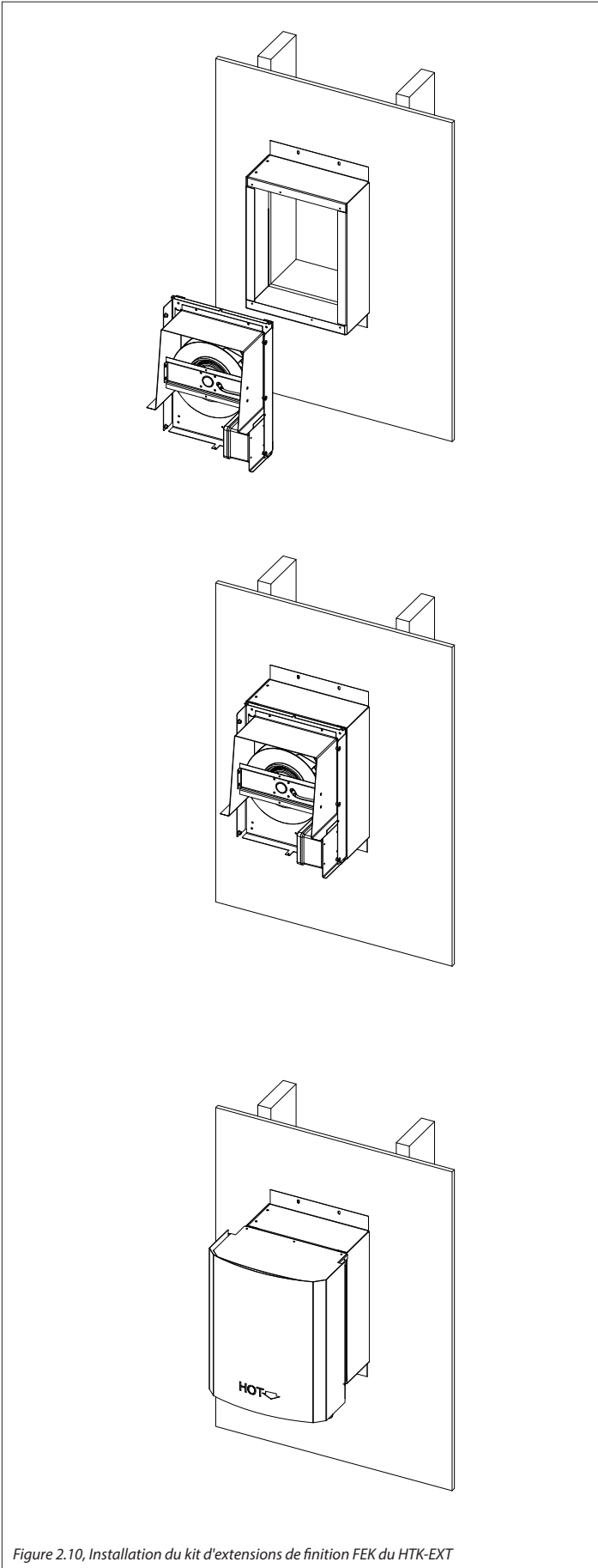
Figure 2.10, Installation du kit d'extensions de finition FEK du HTK-EXT
