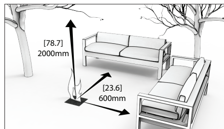
Distanza esterna
