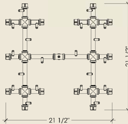
TOP ELEVATION
