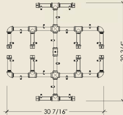
TOP ELEVATION
