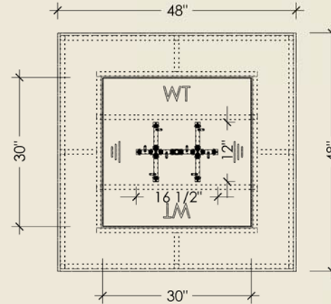
TOP ELEVATION
